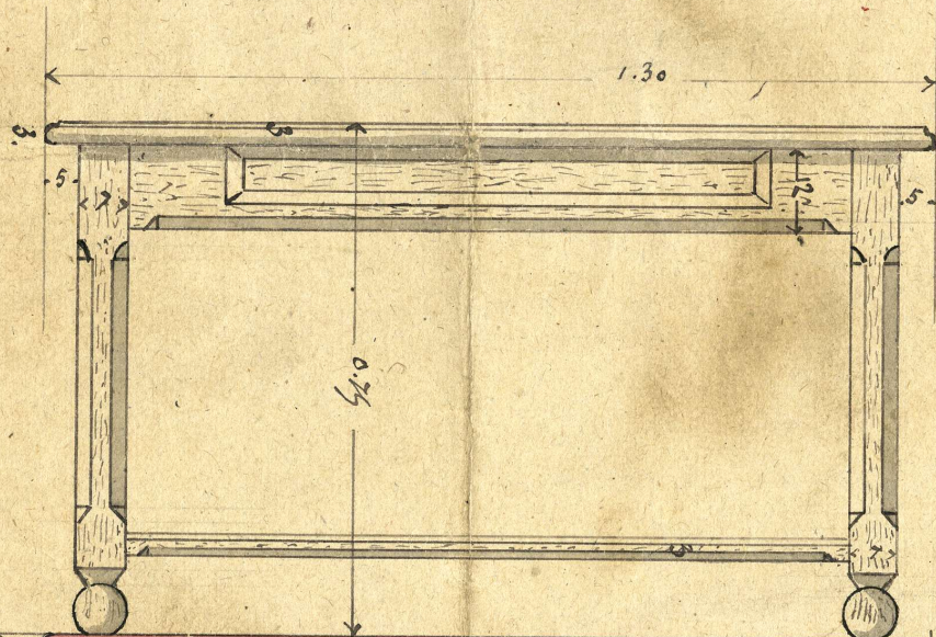
Elevation de la table
