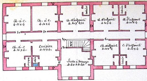
Plan des 2 étages. Logement à l'échelle de 0.05 p. 1 m
